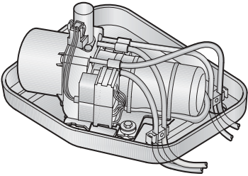
Hydraulikpumpe (mit Umschaltrelais)
